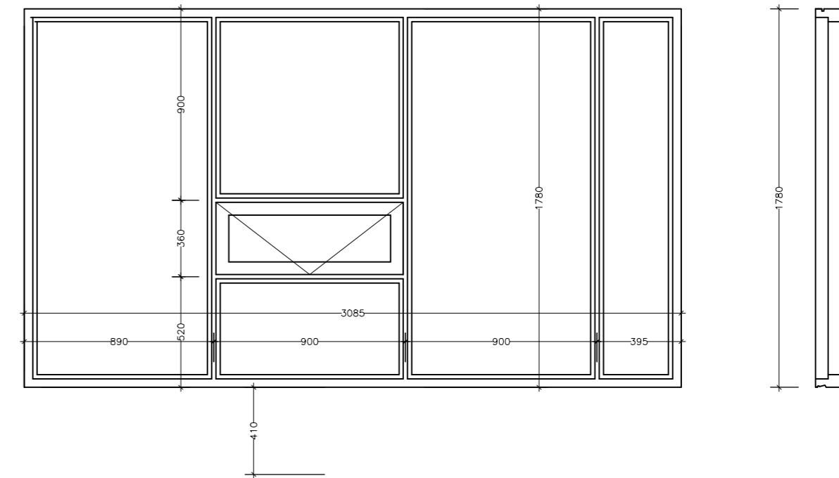
G3 1 stk. (gafi) fl.mál: 5,49 m 2 ummál: 9,73 m
