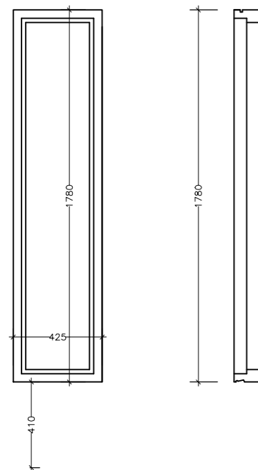
G4 1 stk. (gafi) fl.mál: 0,76 m 2 ummál: 4,41 m
