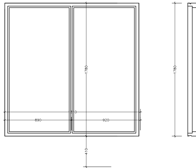
G1 1 stk. fl.mál: 3,19 m 2 ummál: 7,14 m
