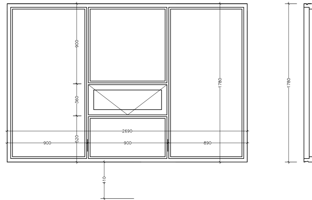
G2 3 stk. fl.mál: 4,79 m 2 ummál: 8,94 m
