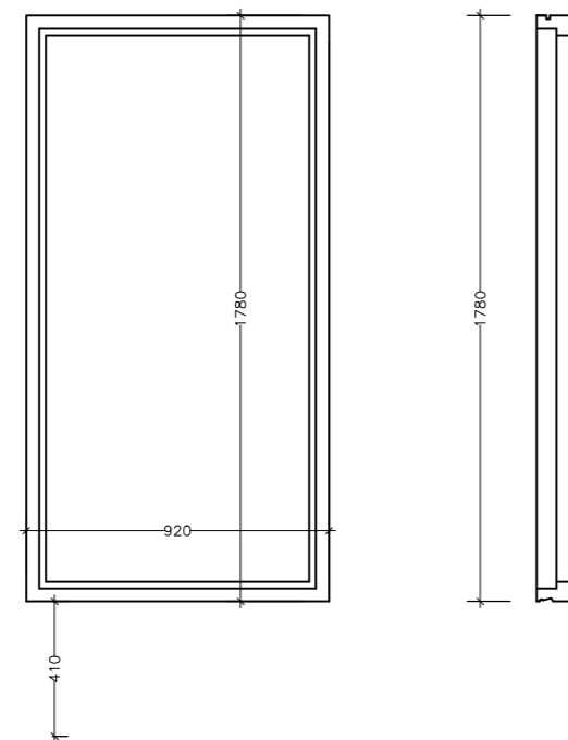
G5 1 stk. (gafi) fl.mál: 1,64 m 2 ummál: 5,40 m
