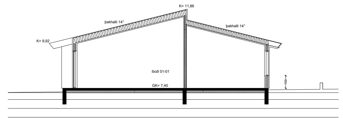
PVERSNIÐ A - A
