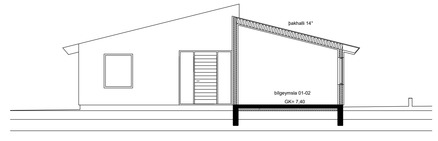
PVERSNIÐ B - B
